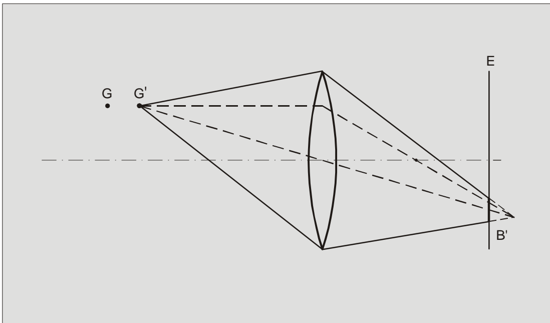
Abb. 11b: Der Punkt wird durch falsche Entfernungseinstellung zu einem Fleck
