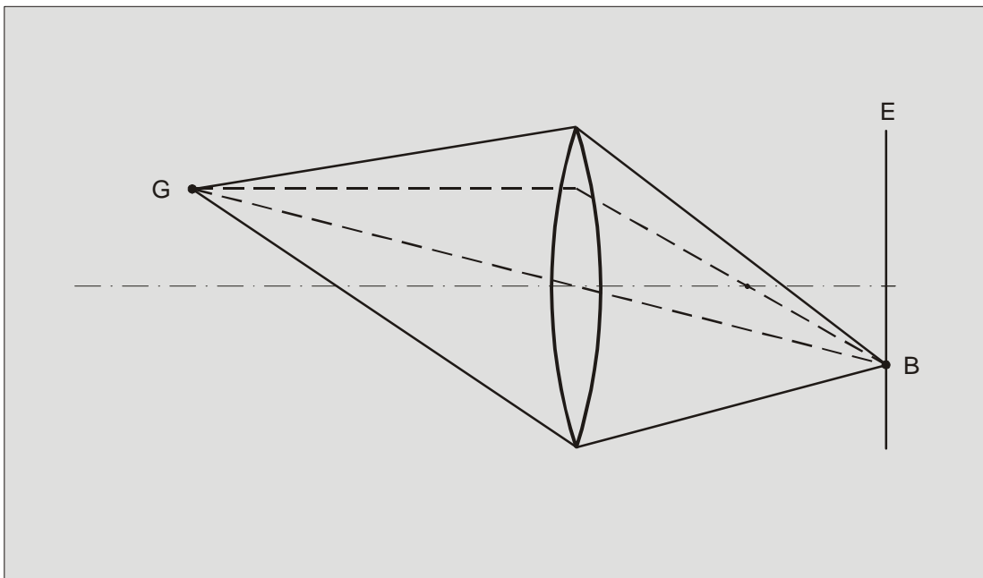
Abb. 11a: Der Bildpunkt in der Filmebene
