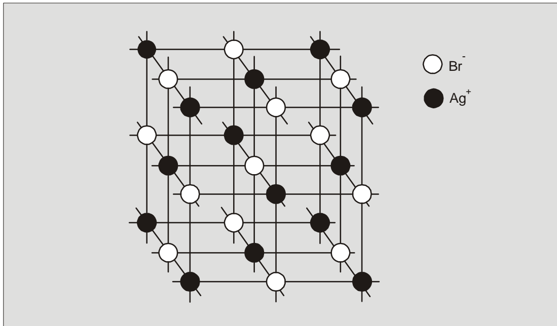
Abb. 16: Das Kristallgitter des Silberbromids
