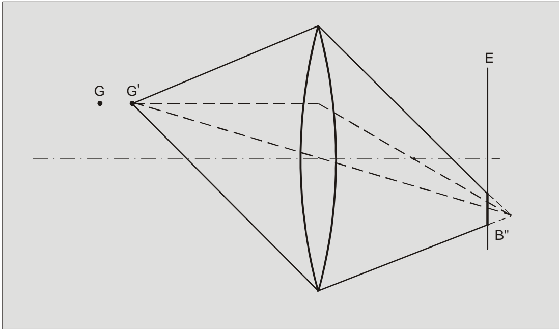
Abb. 11c: Auch durch eine Vergrößerung der Blende wird der Punkt unscharf
