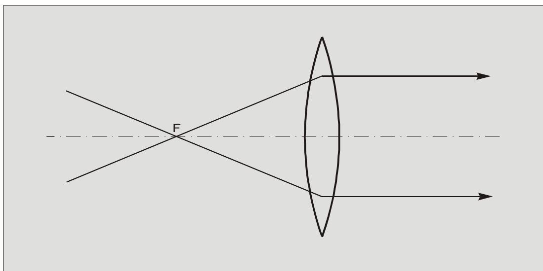
Abb. 2: Brennpunktstrahlen verlassen die Linse als Parallelstrahlen
