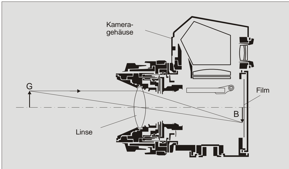
Abb. 5: Prinzip der Abbildung in einer Kamera
