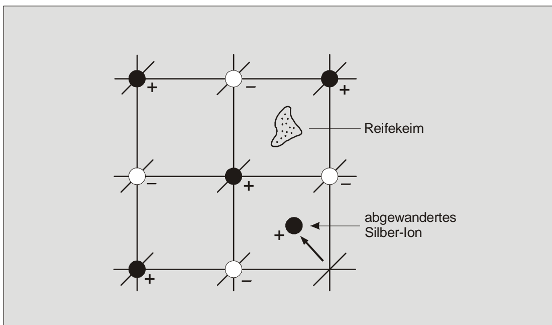
Abb. 17: Freie Gitterplätze und Reifekeime
