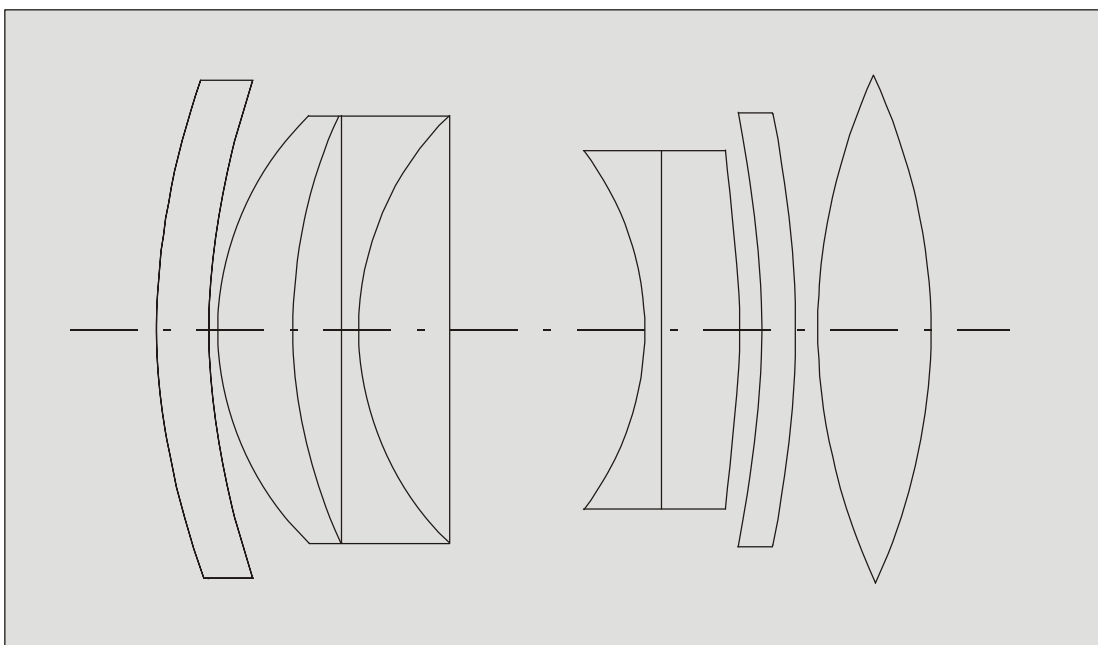
Abb. 8: Linsensystem eines Objektivs
