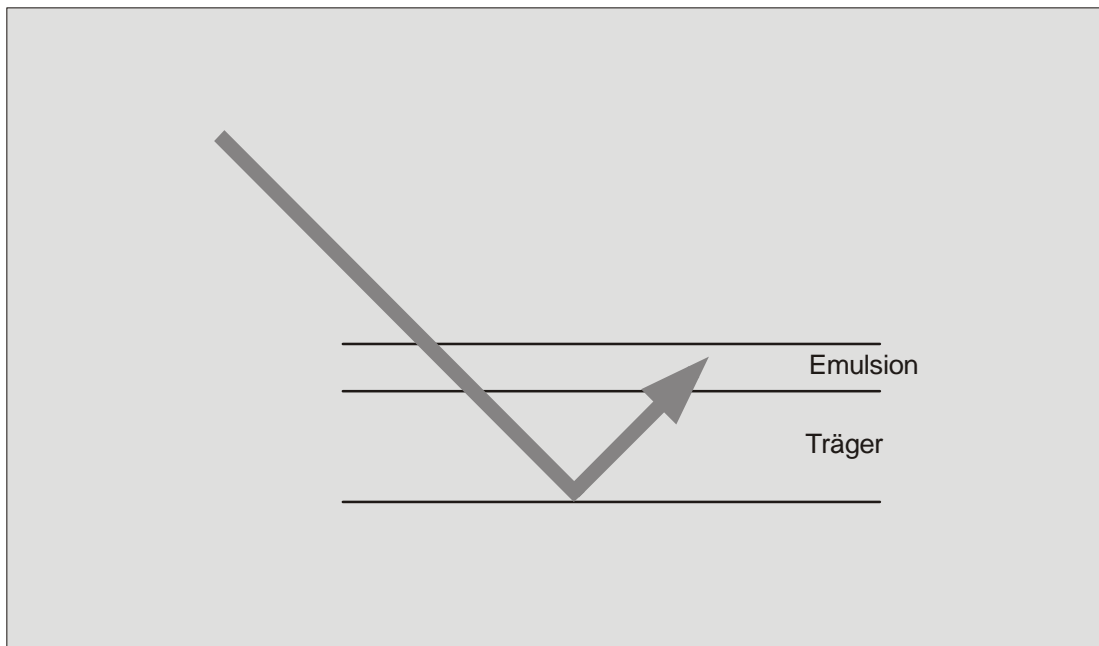
Abb. 13: Unerwünschte Reflexion innerhalb des Films ("Lichthof")
