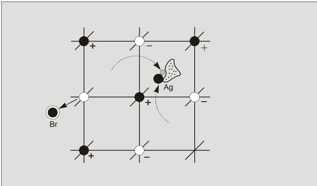
Abb. 19: Am Reifekeim entsteht elementares Silber
