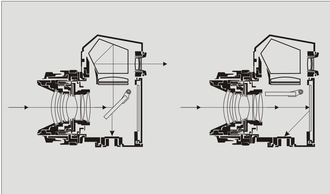
Abb. 9: Spiegelreflexkamera
