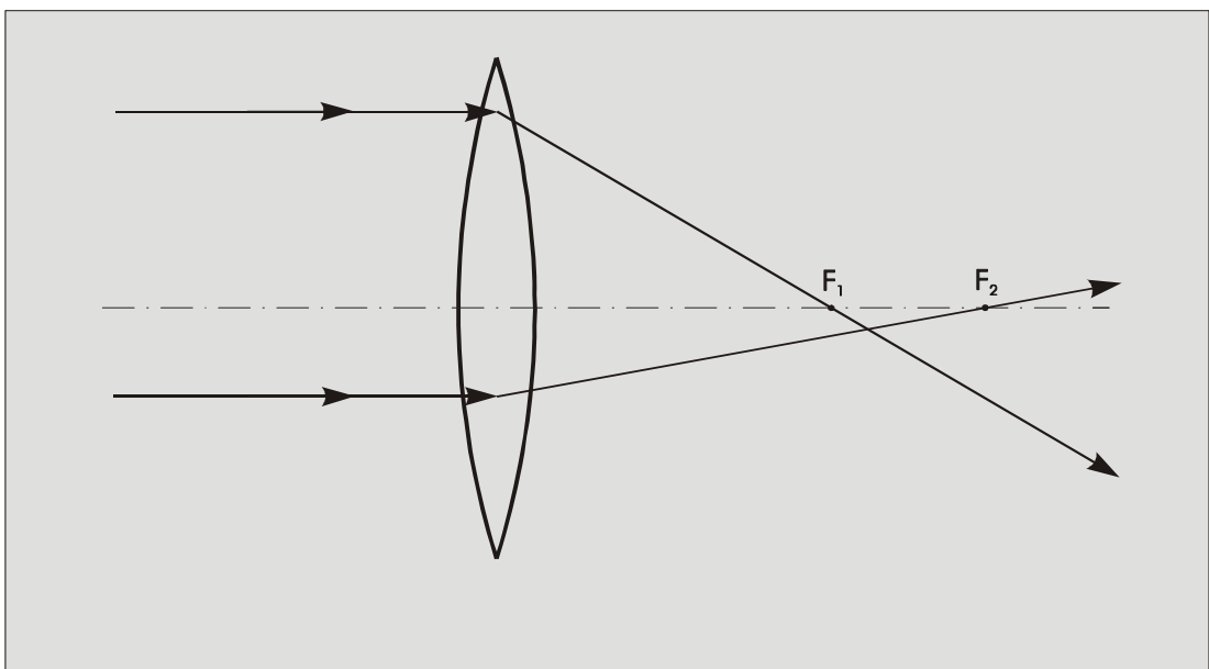
Abb. 6: Sphärische Aberration
