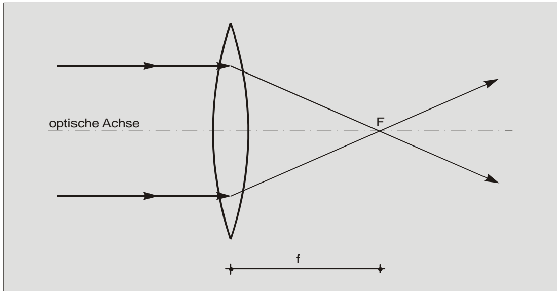
Abb. 1: Brennpunkt und Brennweite
