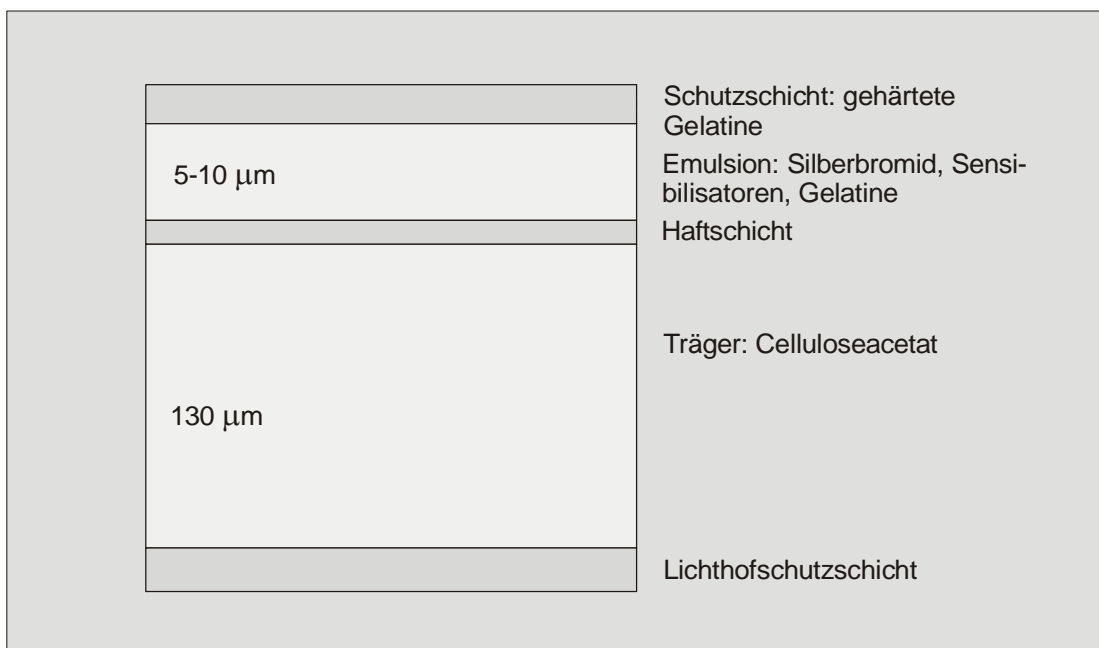
Abb. 14: Aufbau eines Schwarzweißfilms
