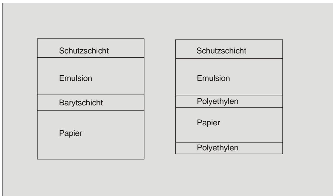
Abb. 15: Barytpapier und PE-Papier
