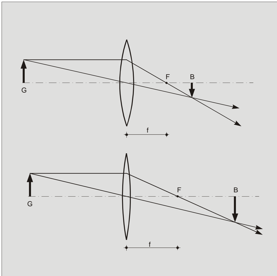
Abb. 10: Die Brennweite bestimmt die Größe des Bildes
