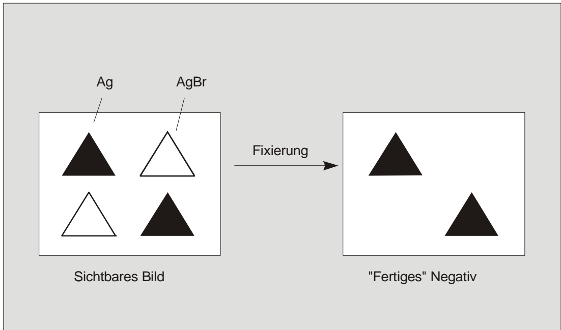
Abb. 21: Restliches Silberbromid wird beim Fixieren entfernt
