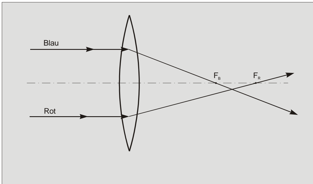
Abb. 7: Chromatische Aberration
